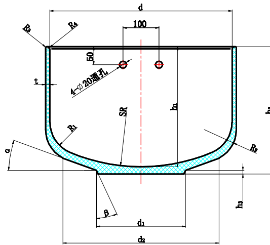
附图一：整体式坩埚
