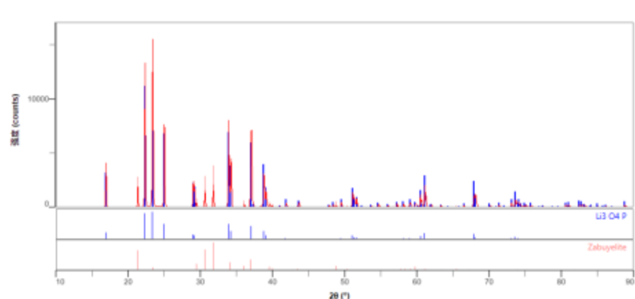
图 2 含量为 95%的磷酸锂 XRD 测试结果
