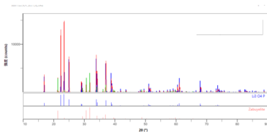
图 4 含量为 85%的磷酸锂 XRD 测试结果
