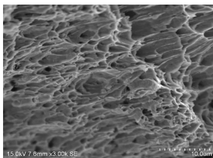
(c) 1300°C高温拉伸断口形貌
