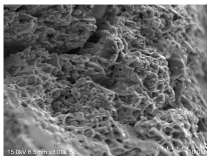
(d) 1400°C高温拉伸断口形貌
