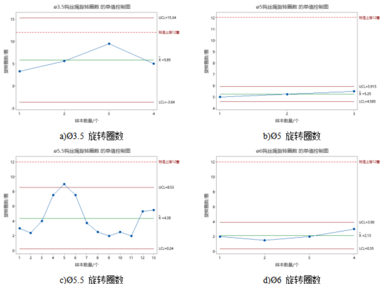
图6 钨丝绳旋转圈数的单值控制图
