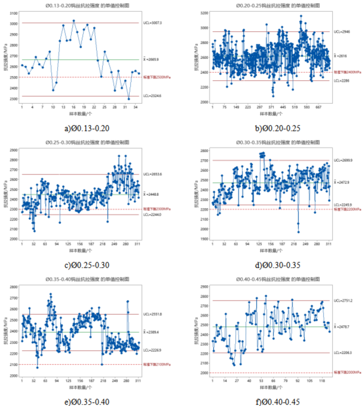
图 1 不同规格钨丝的抗拉强度
