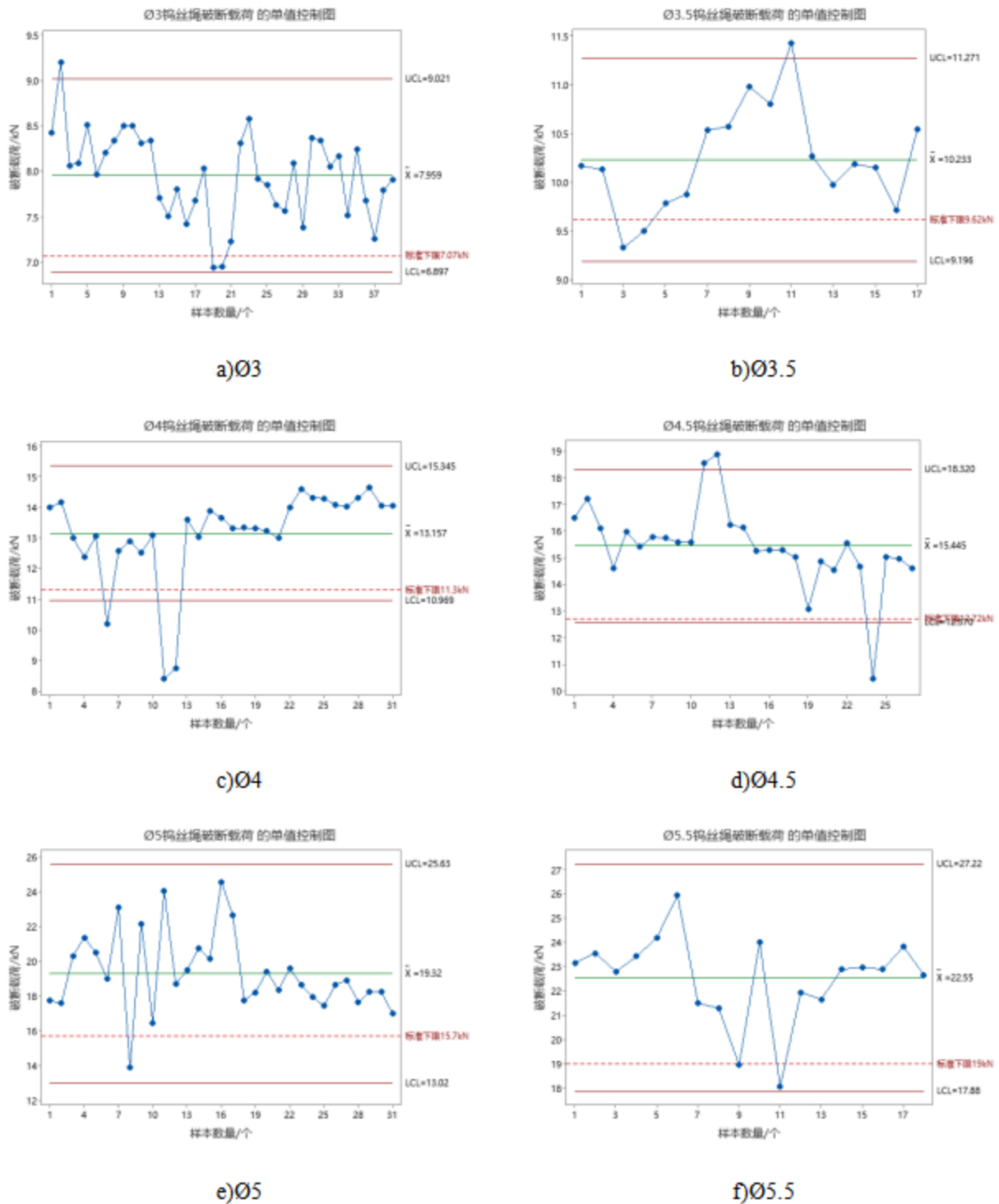
图3 不同规格钢丝绳破断载荷数据分析（室温）
