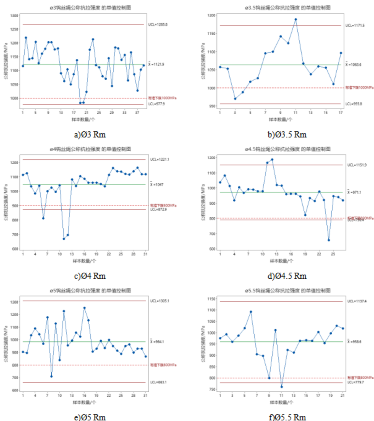
图2 不同规格钢丝绳公称抗拉强度数据分析(室温)
