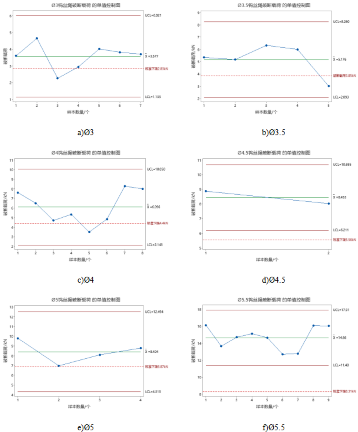
图5 不同规格钢丝绳破断载荷数据分析（高温）
