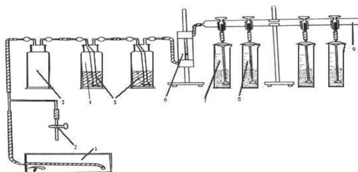
1—无油气体压缩机；2—二通玻璃活塞；3—安全瓶；4—洗气瓶(500 mL)；5—重铬酸钾-硫酸洗涤液； 6—空气流量计(10 L/min~15 L/min)；7—高型烧杯（100 mL）；8—吹气管，末端有6个小孔；9—玻璃管（ \Phi 20 mm）
