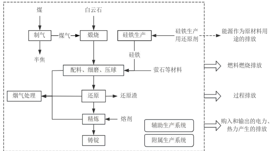
图1 工业硅生产企业温室气体排放核算边界示意图
