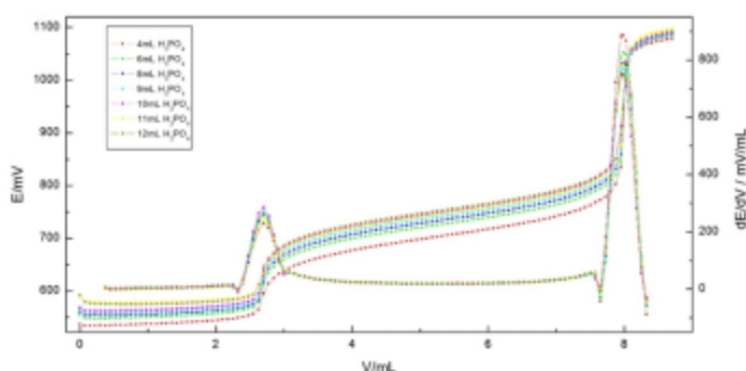
图 2 不同磷酸加入量电位滴定曲线
