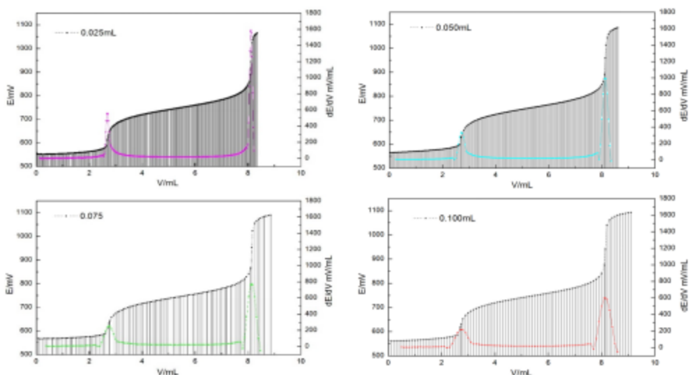
图 1 “滴定体积”不同设定值电位滴定曲线
