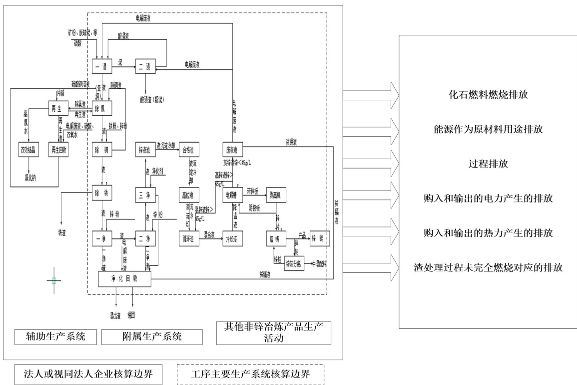
图A.2 湿法炼锌工艺温室气体排放核算边界示意图
