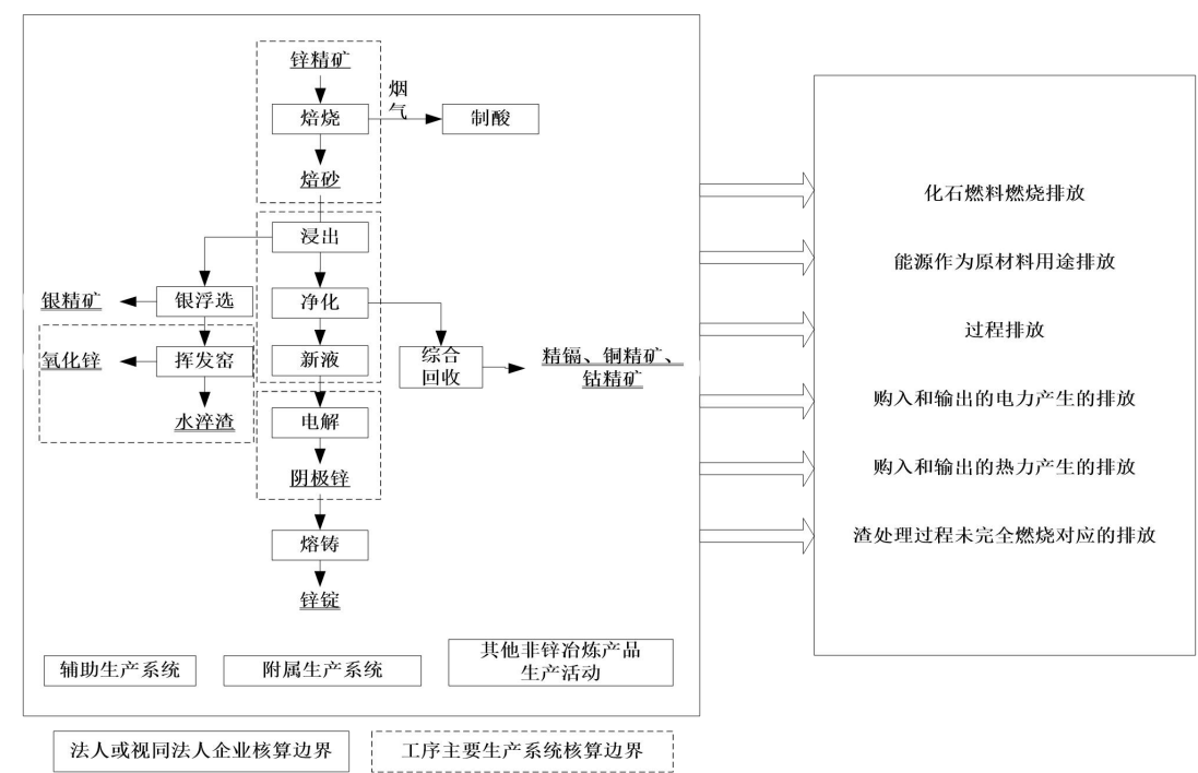
图A.2 湿法炼锌工艺温室气体排放核算边界示意图
