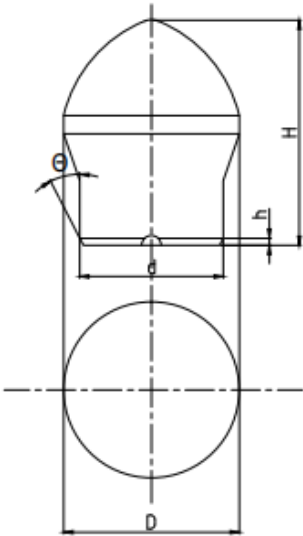
图 2 蘑菇型工程齿示意图
