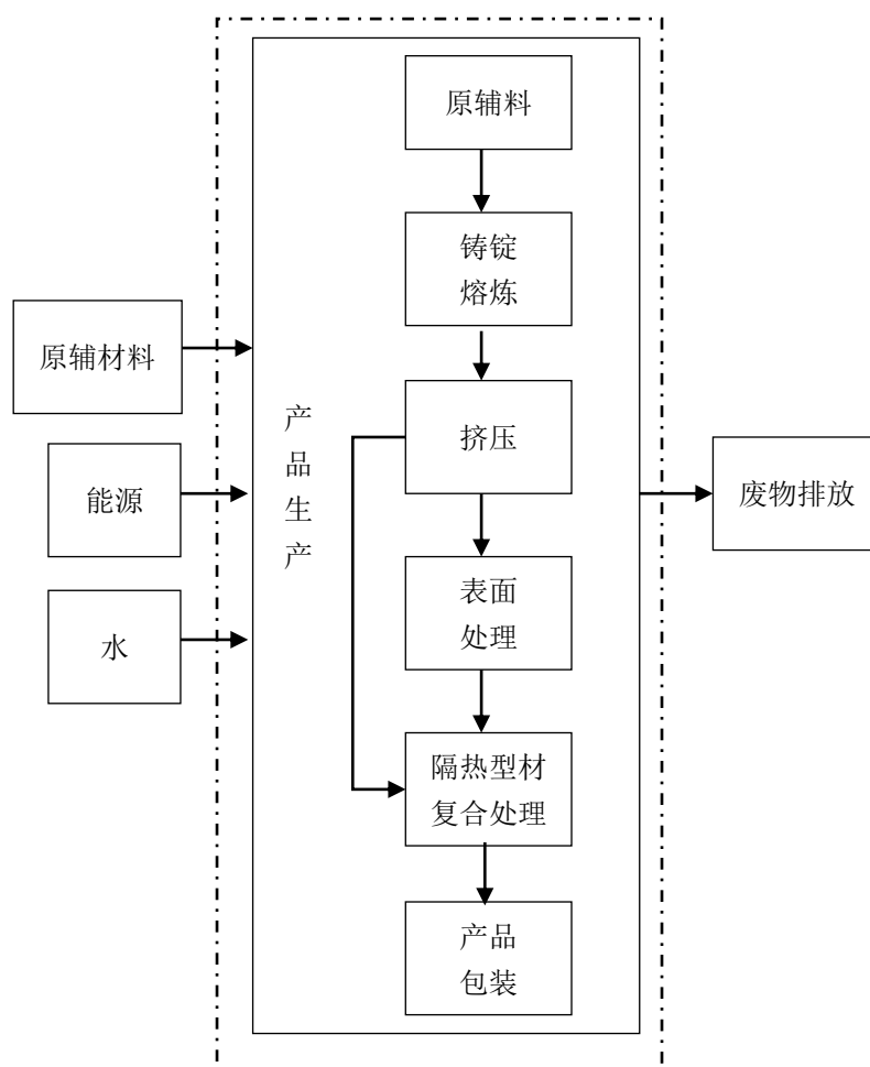
图 B.1 铝合金建筑型材产品系统边界图
