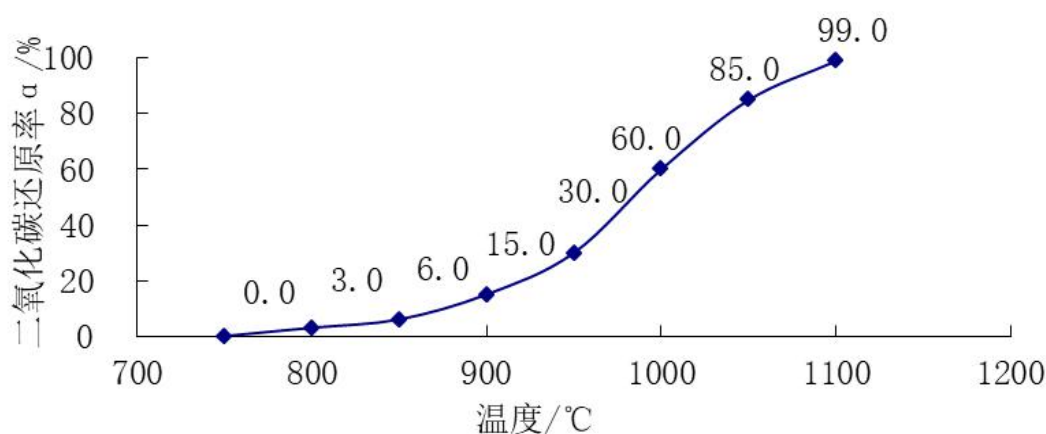
图 1 洁净炭的二氧化碳反应曲线
